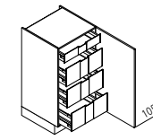
VI Larder unit ↔ 40/45/50/60 ↓ 105 ↖ 60/50/35
